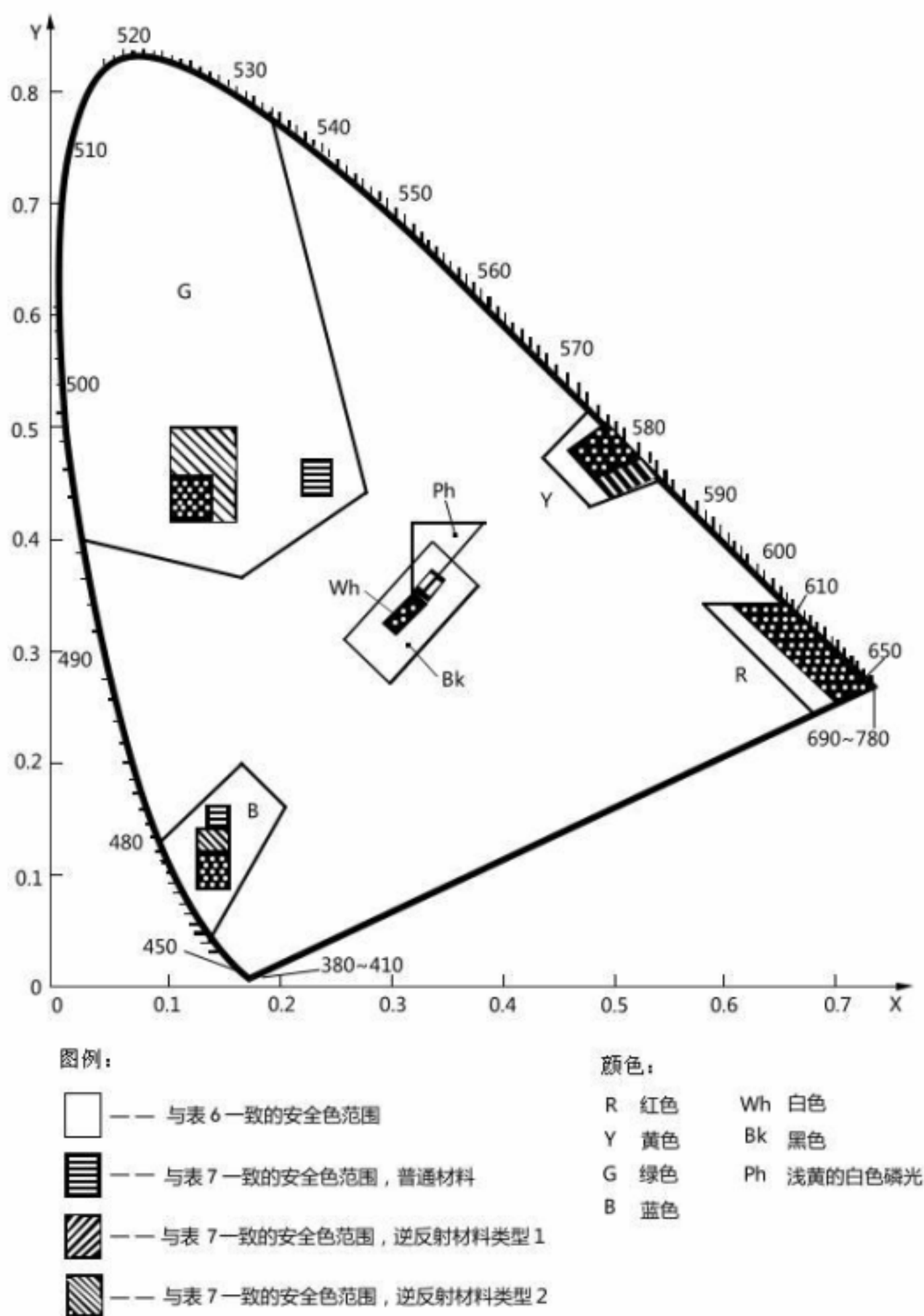
图 1 安全色和对比色的色品区域图
