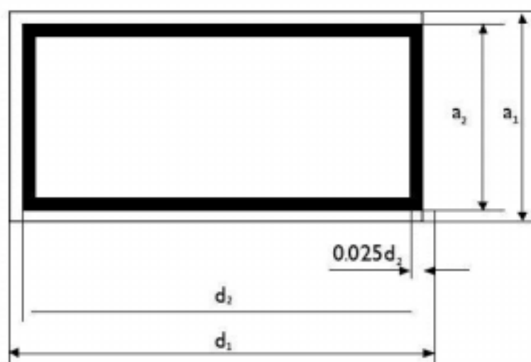
图A.5 附加提示标识基本型式
