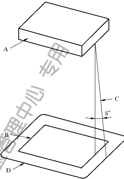
图 6 挡板
