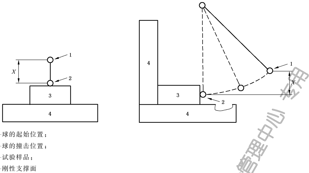
图 4 使用钢球的撞击试验
